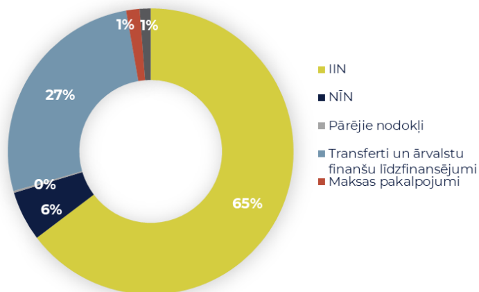
Ieņēmumi, 2025.g. (%)
