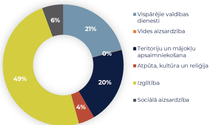
Izdevumi, 2025.g. (%)
