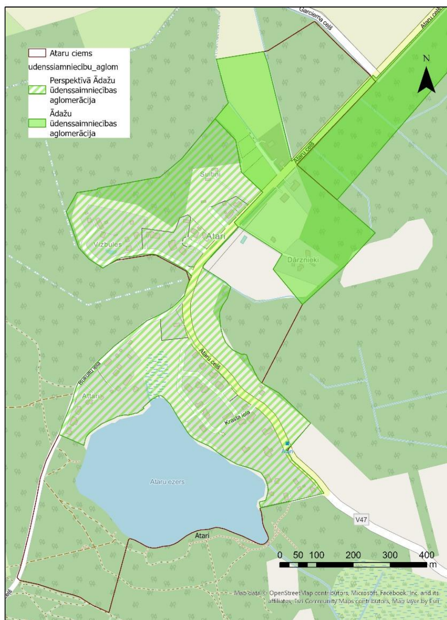
12 attēls Ataru ciemā esošā un plānotā ūdenssaimniecības aglomerācija
