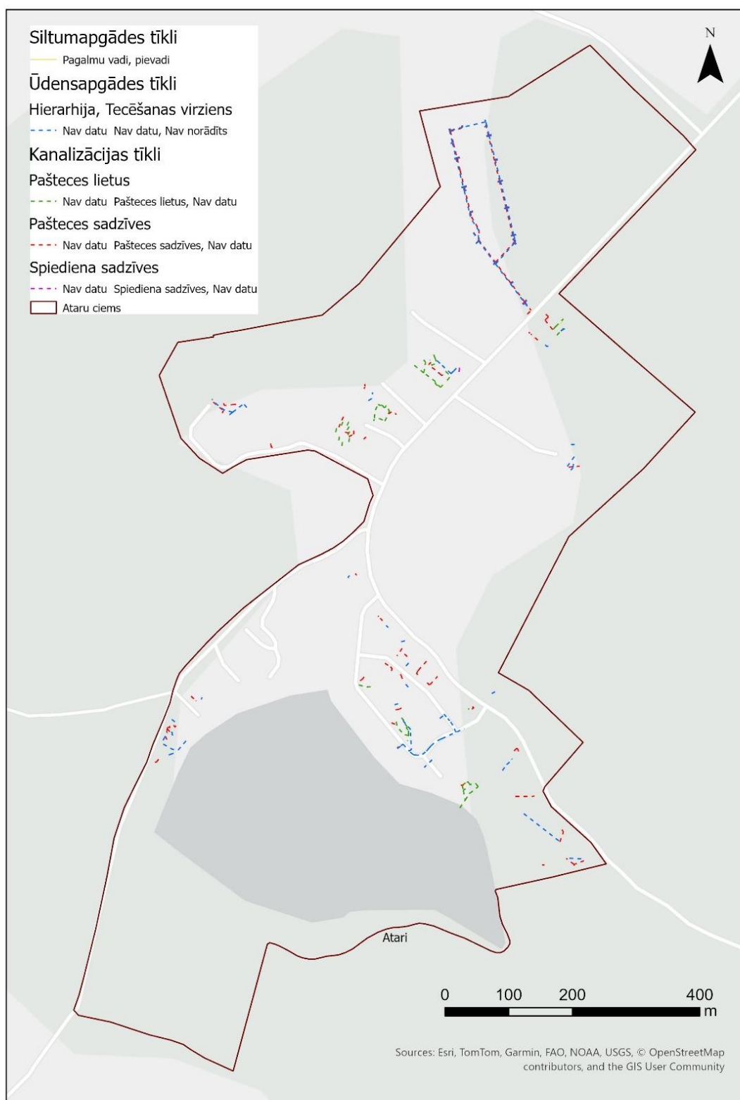
11 attēls Ataru ciema tehniskā infrastruktūra
