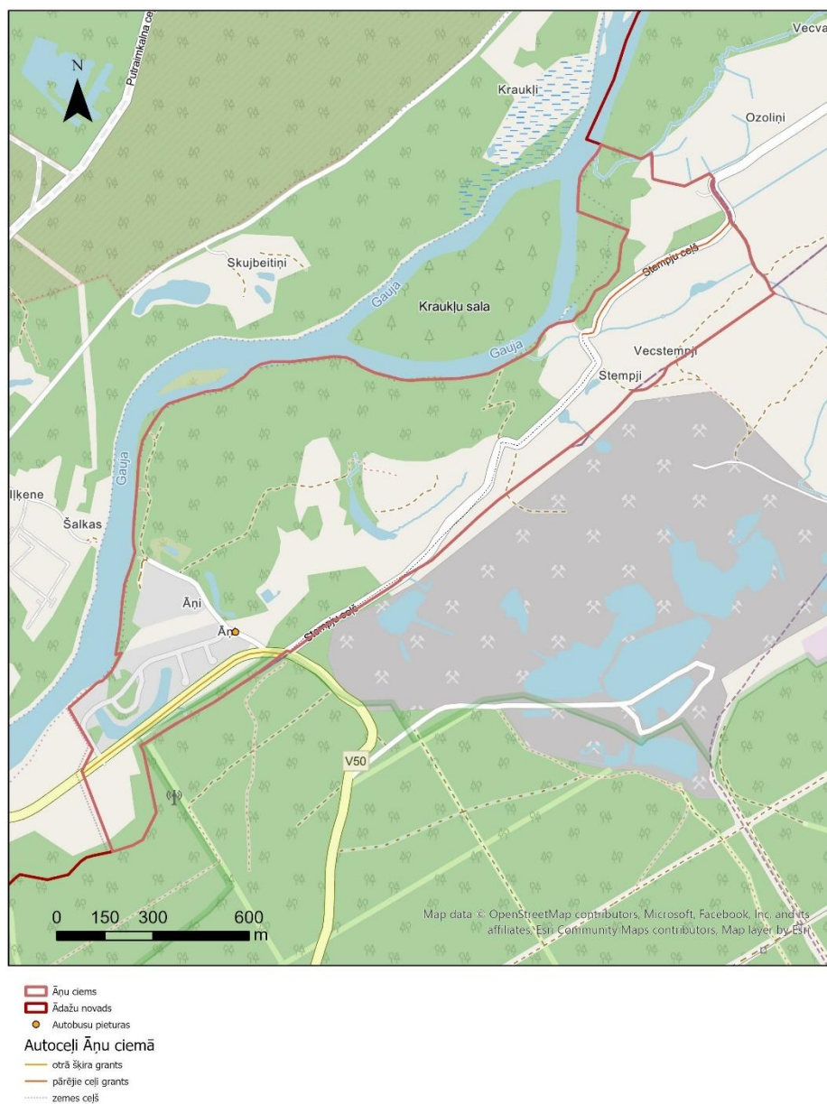
9 attēls Āņu ciema transporta infrastruktūra
