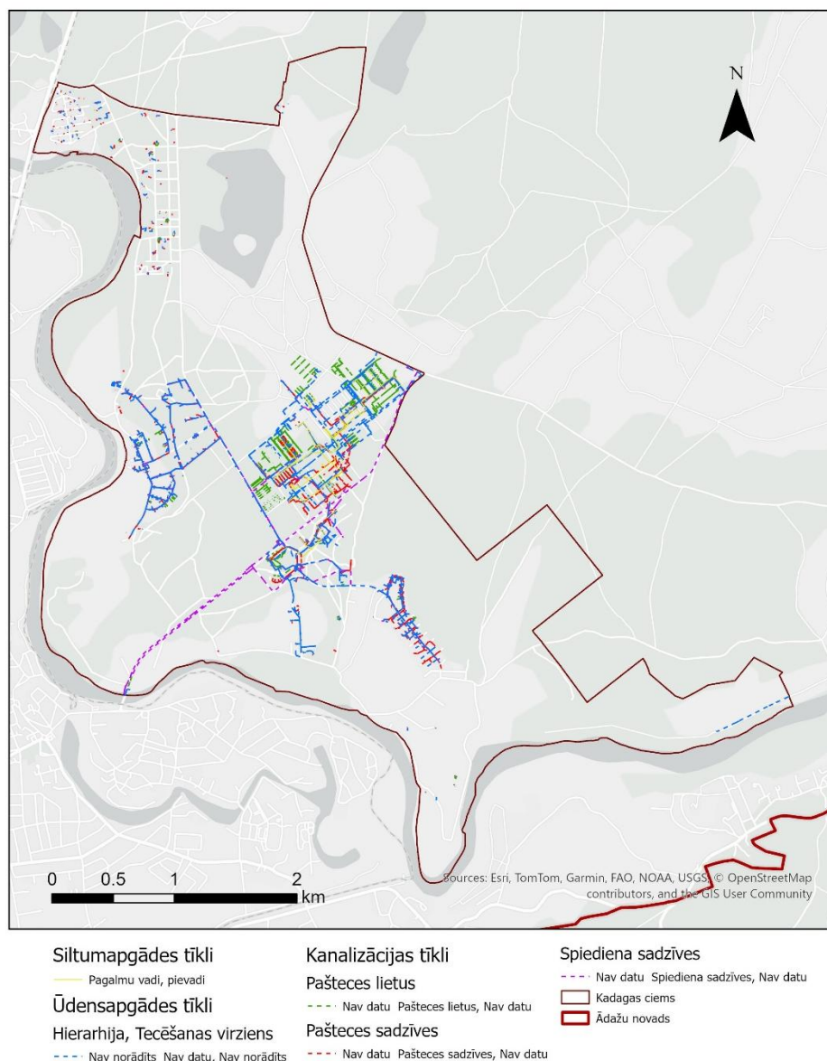
10 attēls Kadagas ciema tehniskā infrastruktūra
