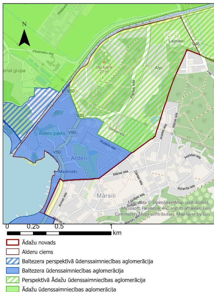
11 attēls Alderu ciemā esošā un plānotā ūdenssaimniecības aglomerācija
