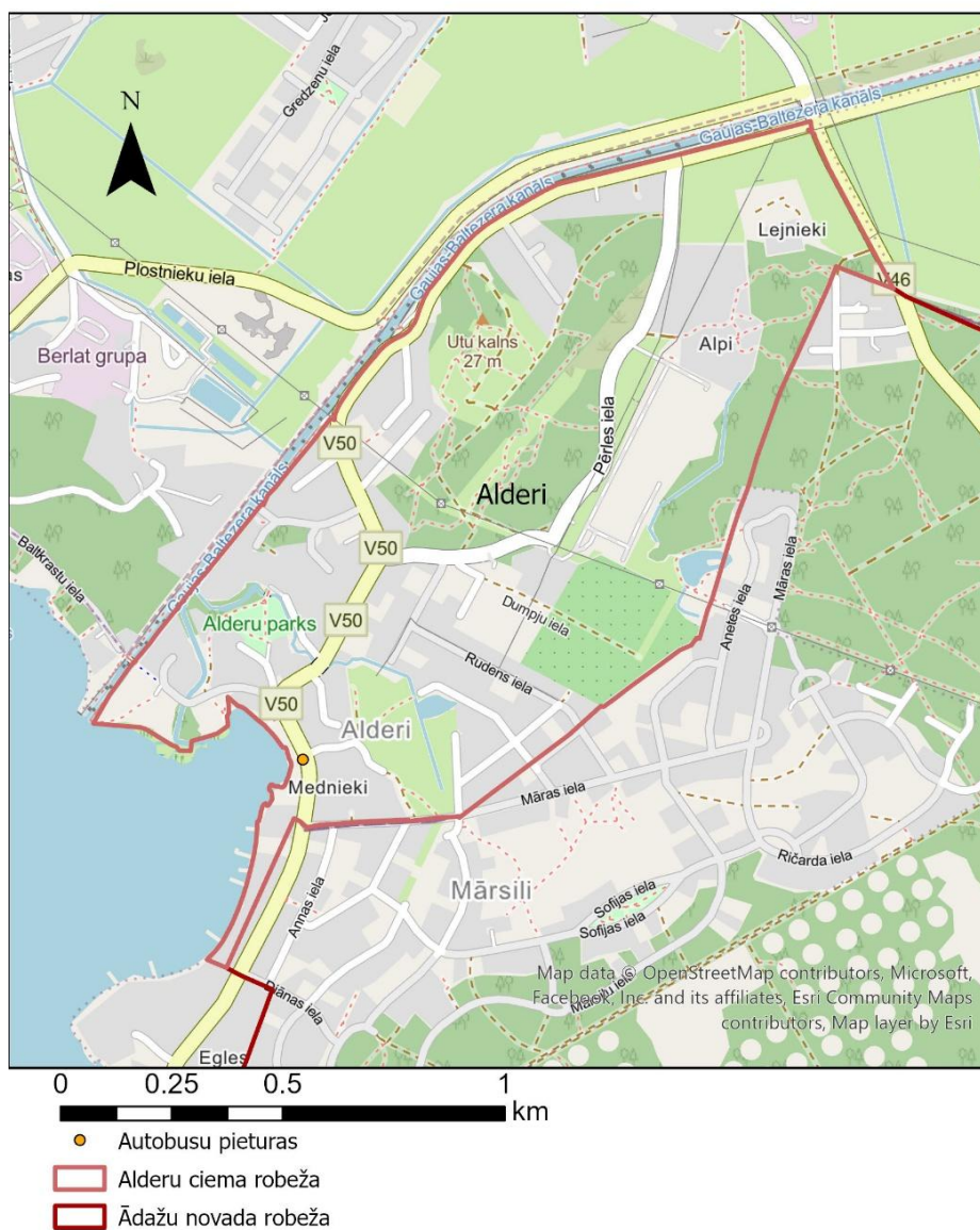
8 attēls Alderu ciema transporta infrastruktūra
