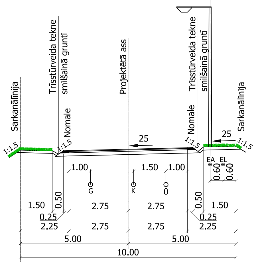
Pamatprofils pie sarkano līniju platuma 10.0m* G-G, M1:100
