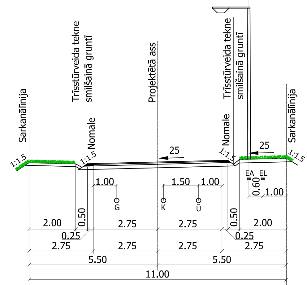
Pamatprofils pie sarkano līniju platuma 11.0m* B-B, C-C, D-D, E-E, F-F, M1:100
