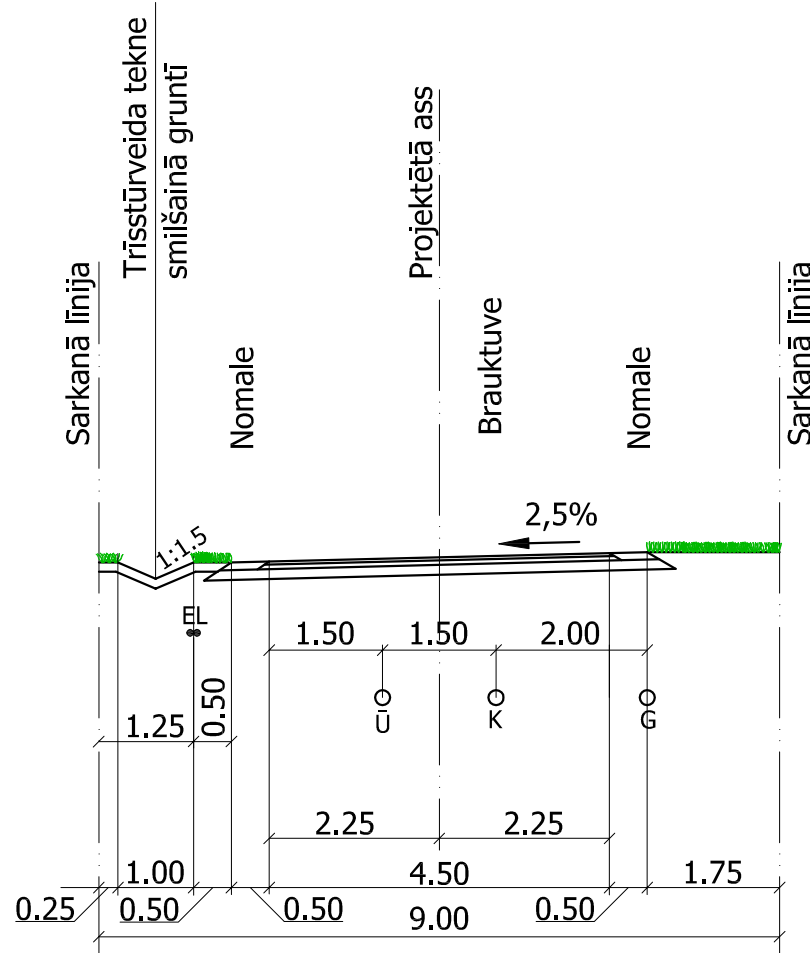
Pamatprofils pie sarkano līniju platuma 9.0m* H-H, I-I, M1:100
