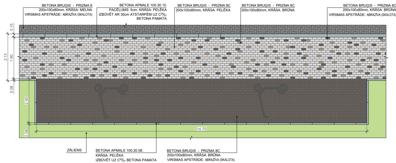
IZKLĀJUMS NR.4 (SKRERITEŅU NOVIETNE)
