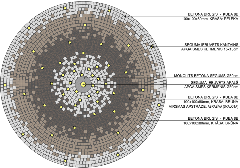
IZKLĀJUMS NR.5 (ATPŪTAS ZONA)
