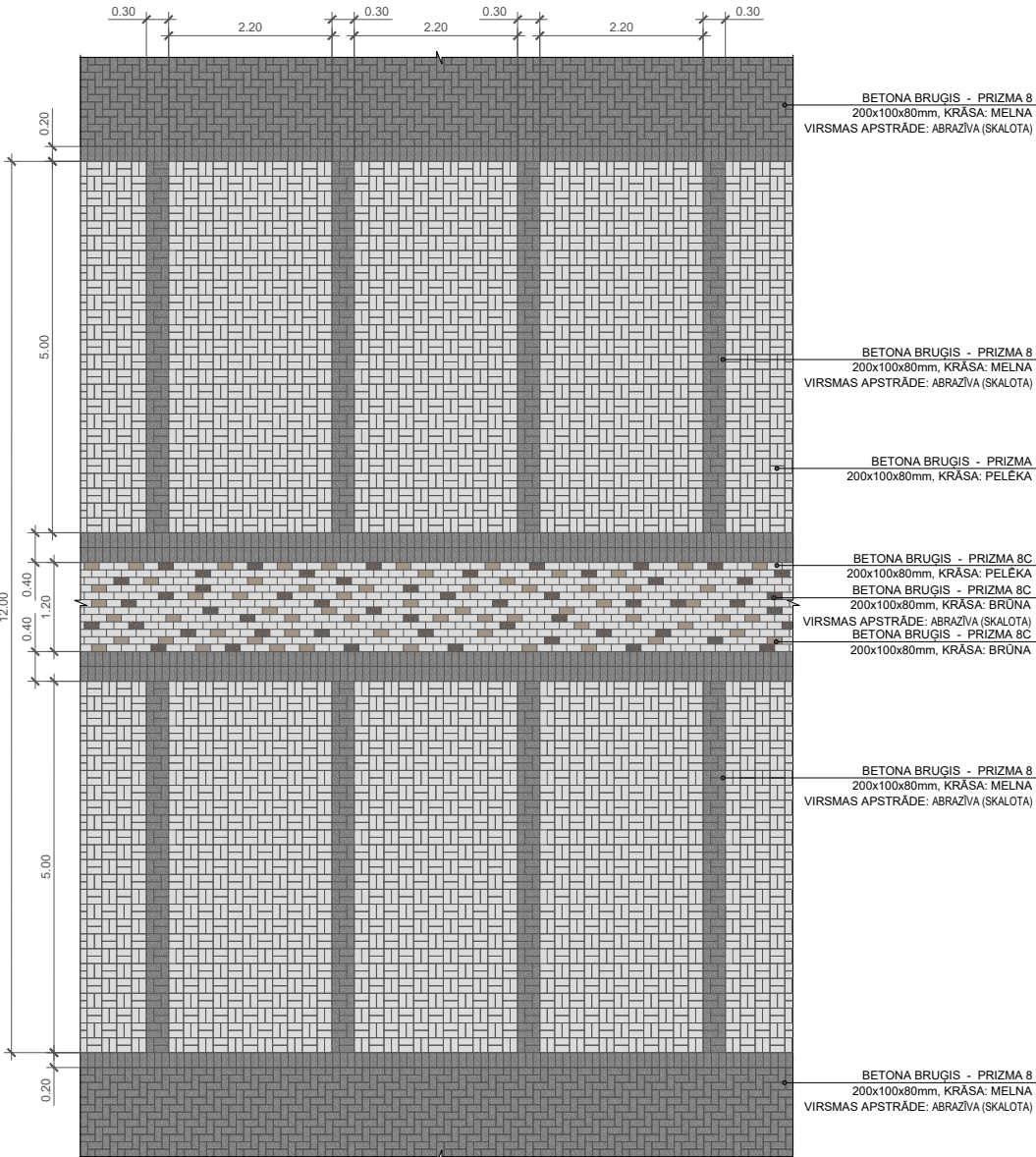
IZKLĀJUMS NR.2 (STĀVVIETAS LAUKUMA CENTRĀ)
