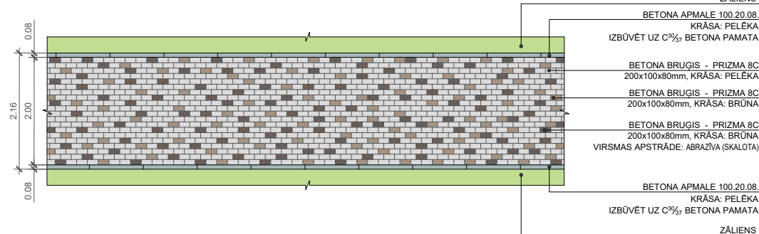
IZKLĀJUMS NR.3 (IETVES)
