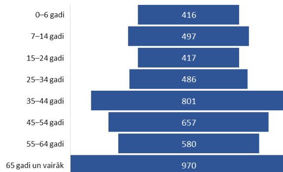
7 attēls Iedzīvotāju skaits Carnikavas ciemā vecuma grupās, 01.01.2024. (Info: CSP)
