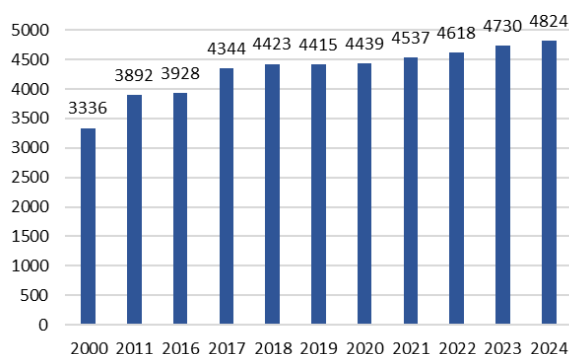
5 attēls Iedzīvotāju skaita izmaiņas Carnikavas ciemā 2000.-2024., uz gada sākumu (Info: CSP)
