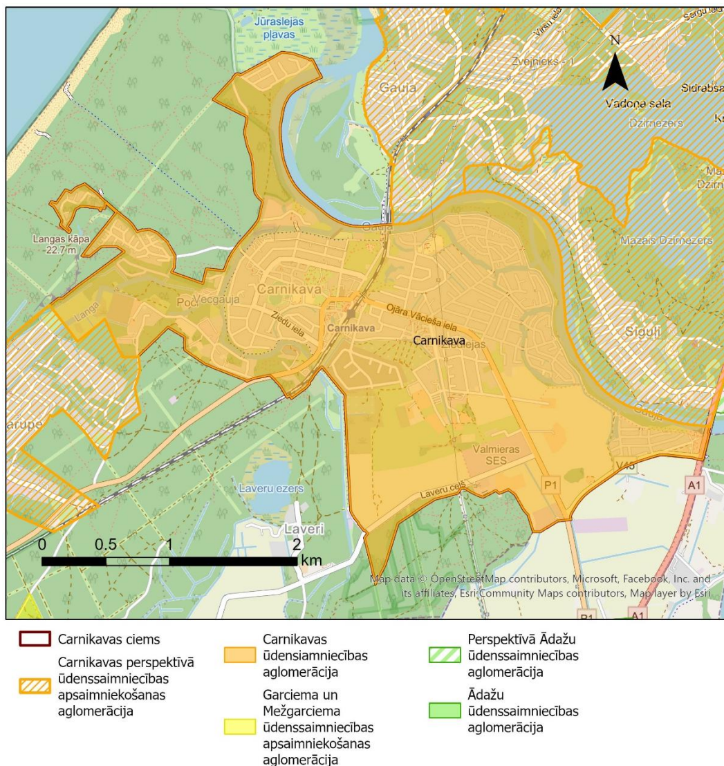
11 attēls Carnikavas ciemā esošā un plānotā ūdenssaimniecības aglomerācija
