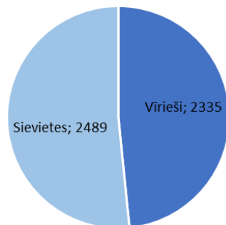
6 attēls Iedzīvotāju skaits Carnikavas ciemā pēc dzimuma, 01.01.2024. (Info: CSP)
