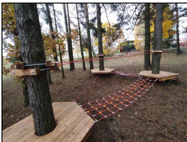
PAPILDINĀTA ESOŠĀ ŠĶĒRŠĻU TAKA AR VIRVJU SIETIEM, LAIPĀM UN PLATFORMĀM
